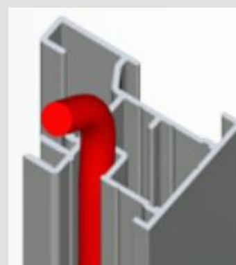
Integrovanie motorového kábla do koľajnice
